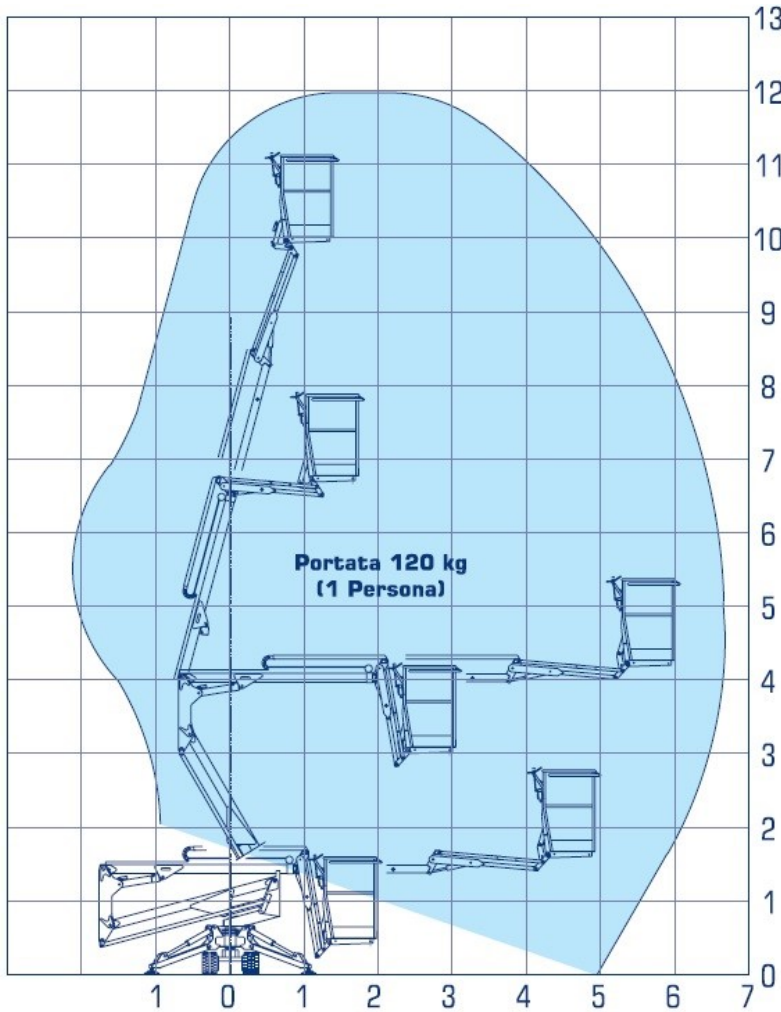
Area di lavoro OCTOPUSSY 1265
